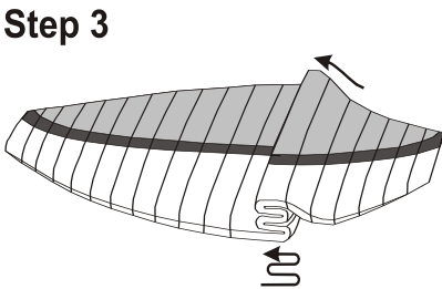
Abbildung 10: Packing the UP Kibo
